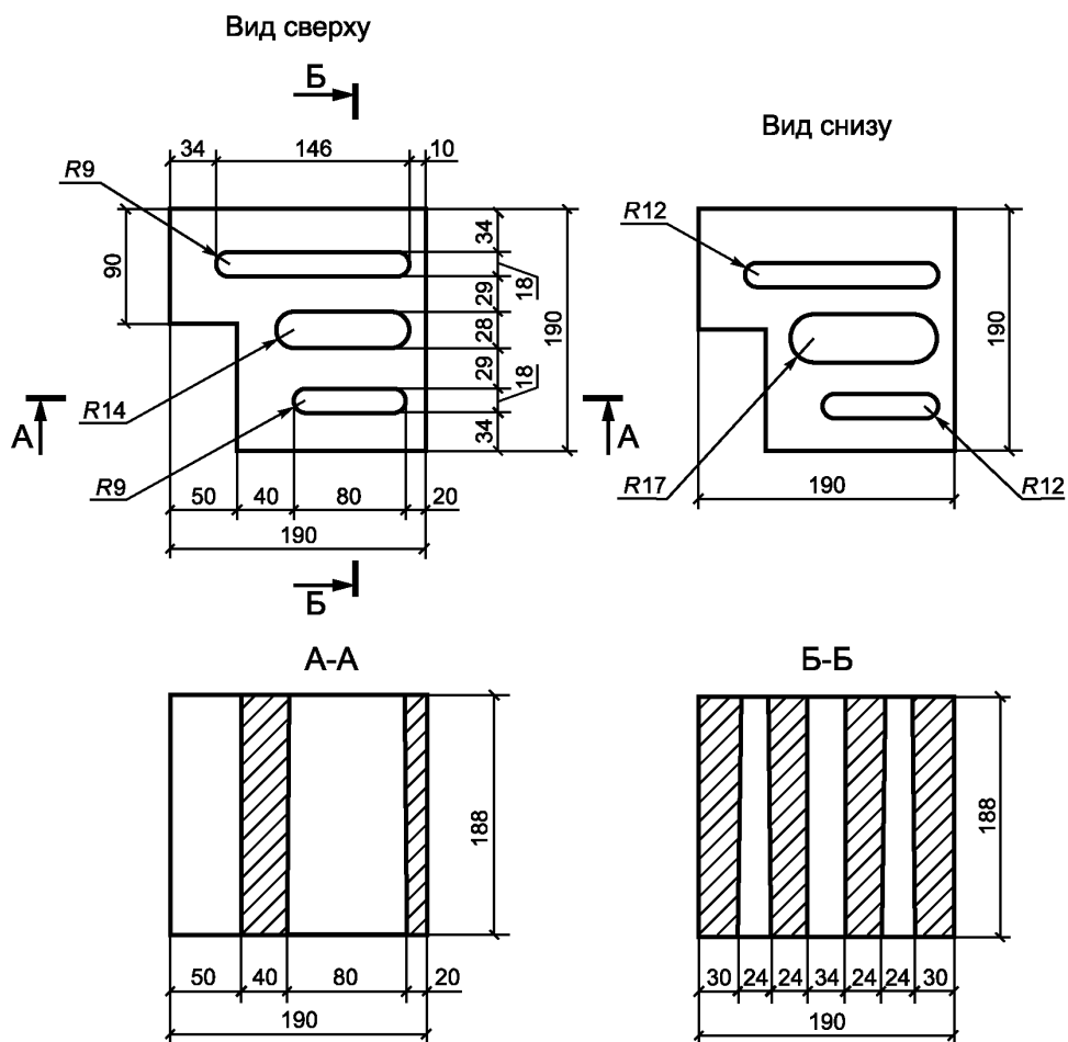
Рисунок А.10 — Камень дополнительный стеновой рядовой (поперечная половинка с четвертью)
