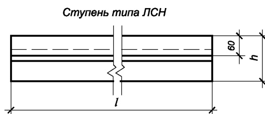
Рисунок 1 — Ступени типоразмеров ЛС, ЛСВ, ЛСП, ЛСН
