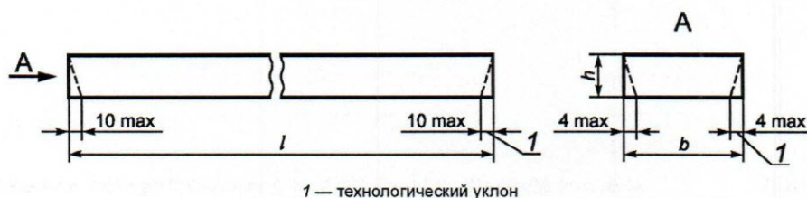
Рисунок 2 — Перемычка типа ПП
