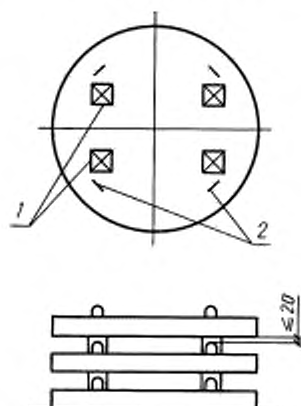
Схема складирования плит перекрытия и дна колодцев
